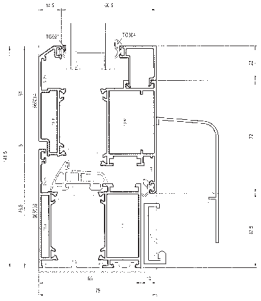
Scorrevole parallelo binario inferiore
