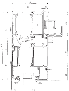
Scorrevole parallelo binario superiore
