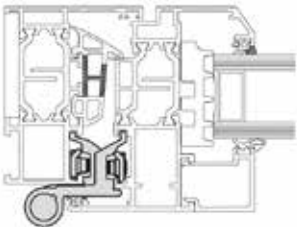
Accessori funzionali CE
